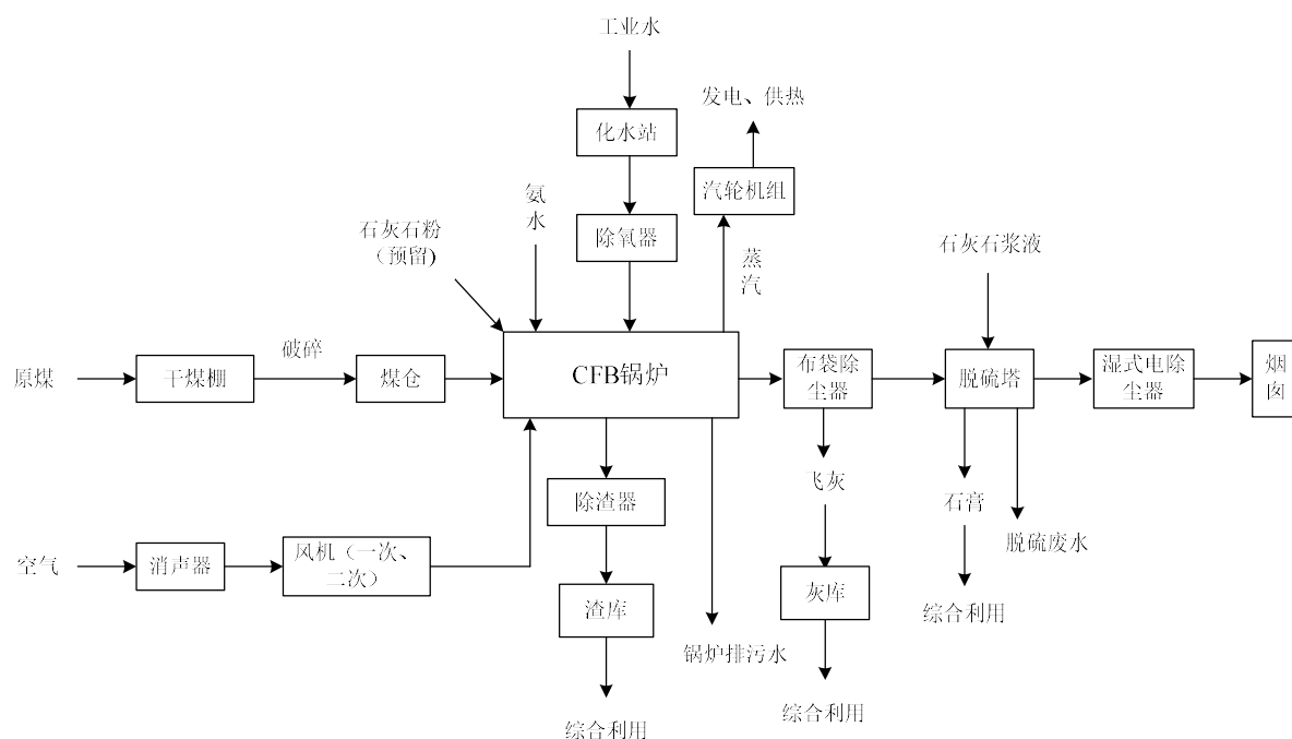
图 3-1 项目工艺流程图
